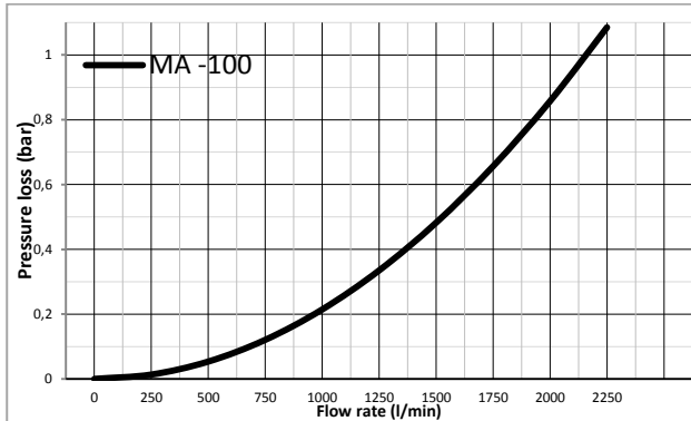
Diagramma perdita di carico - Pressure loss diagram
